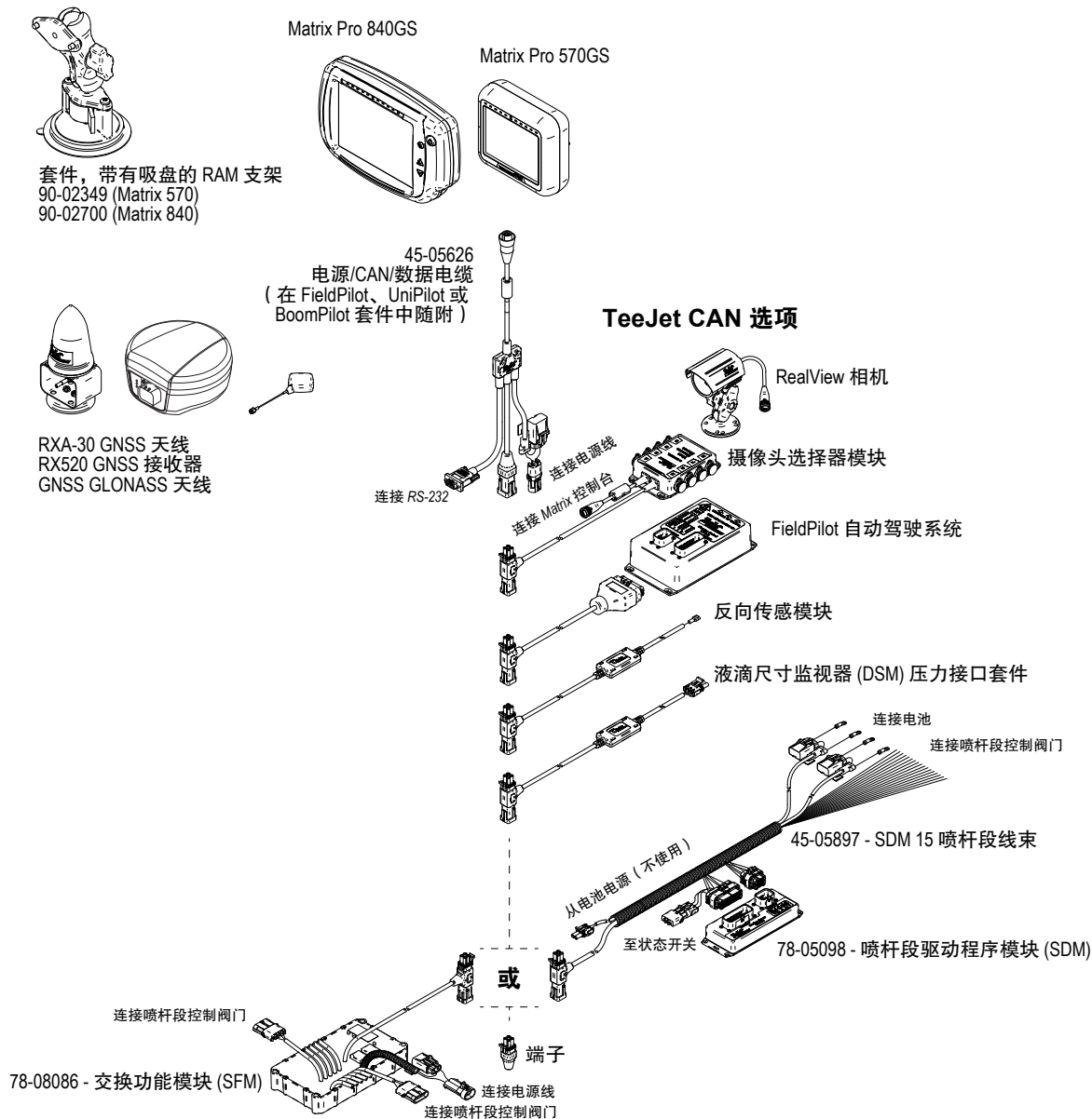
图 A-1: 带 FieldPilot 自动驾驶系统的 Matrix Pro GS
