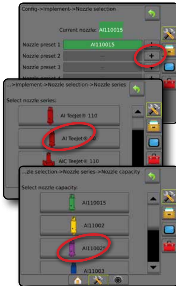
图 6-33: 喷嘴大小和相关颜色
