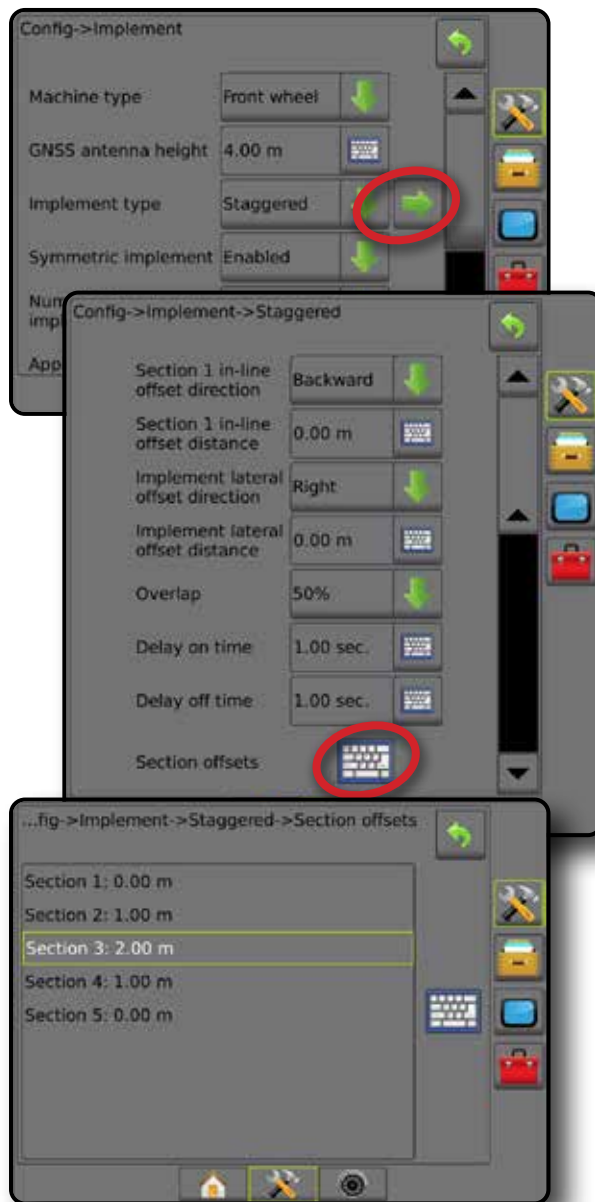
图 6-20: 偏移方向和距离 - 喷杆段 1 之后
