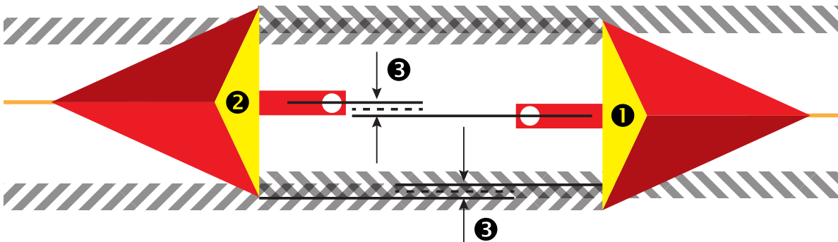
Abbildung 8: GNSS-Versatzabstand
