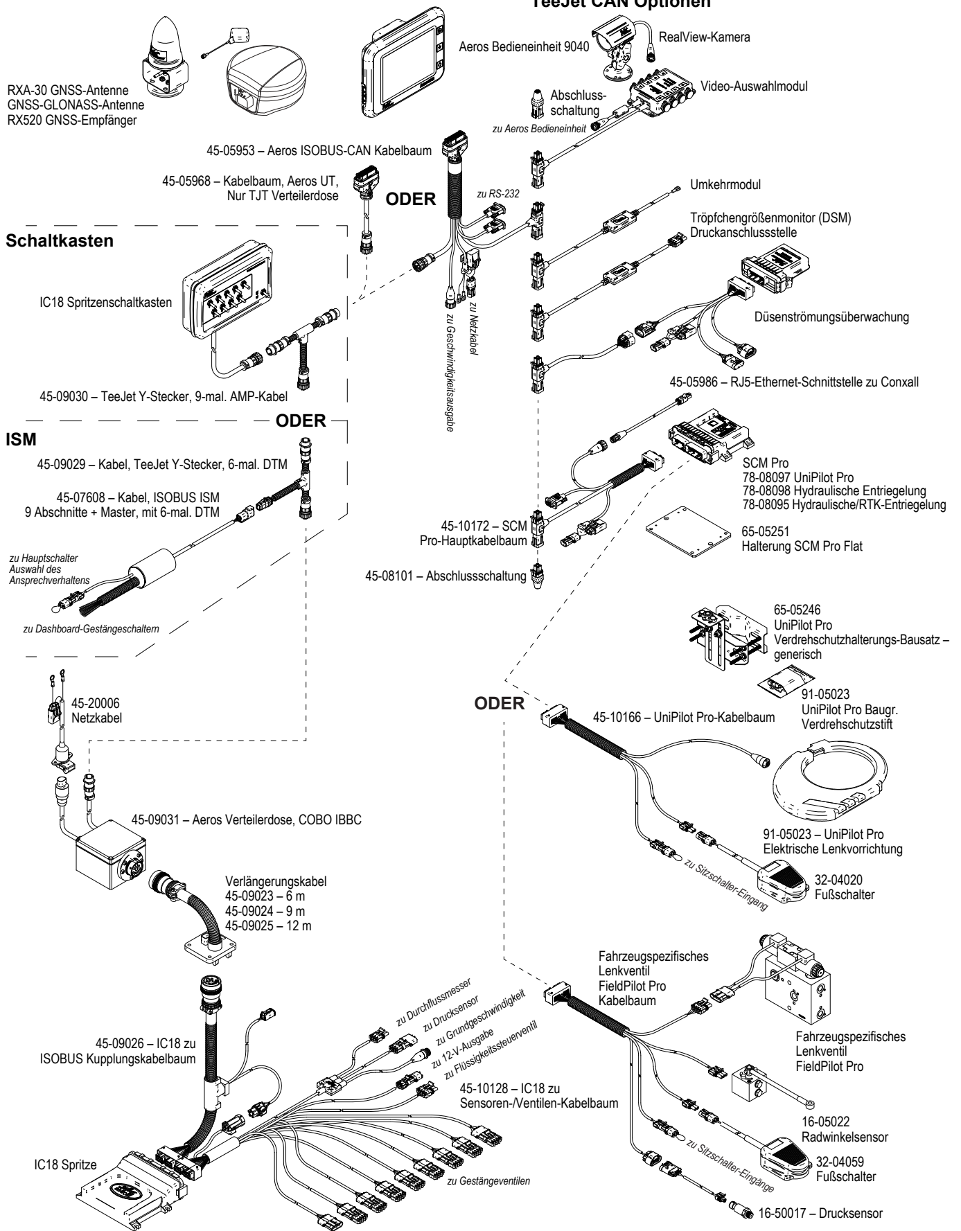
Abbildung 36: Aeros IC18 Spritzen mit FieldPilot Pro oder UniPilot Pro-Lenkssystem
