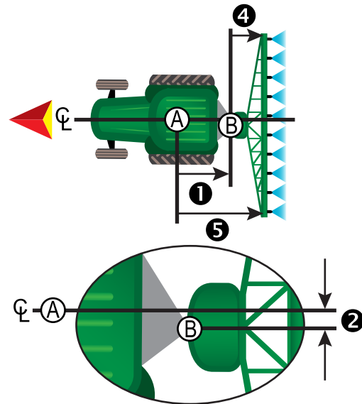
Abbildung 31: Heckmontage
