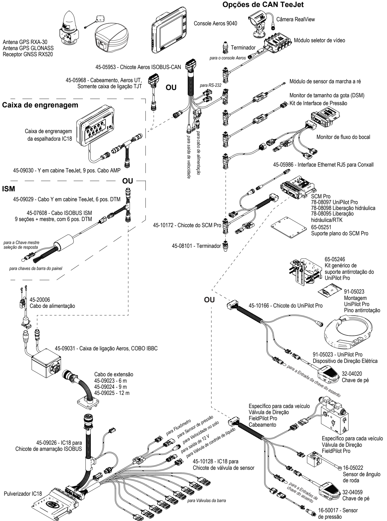
Figura 36: Pulverizador Aeros IC18 com sistema de direção FieldPilot Pro ou UniPilot Pro
