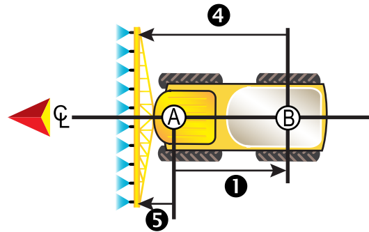
Figura 29: Montagem traseira
