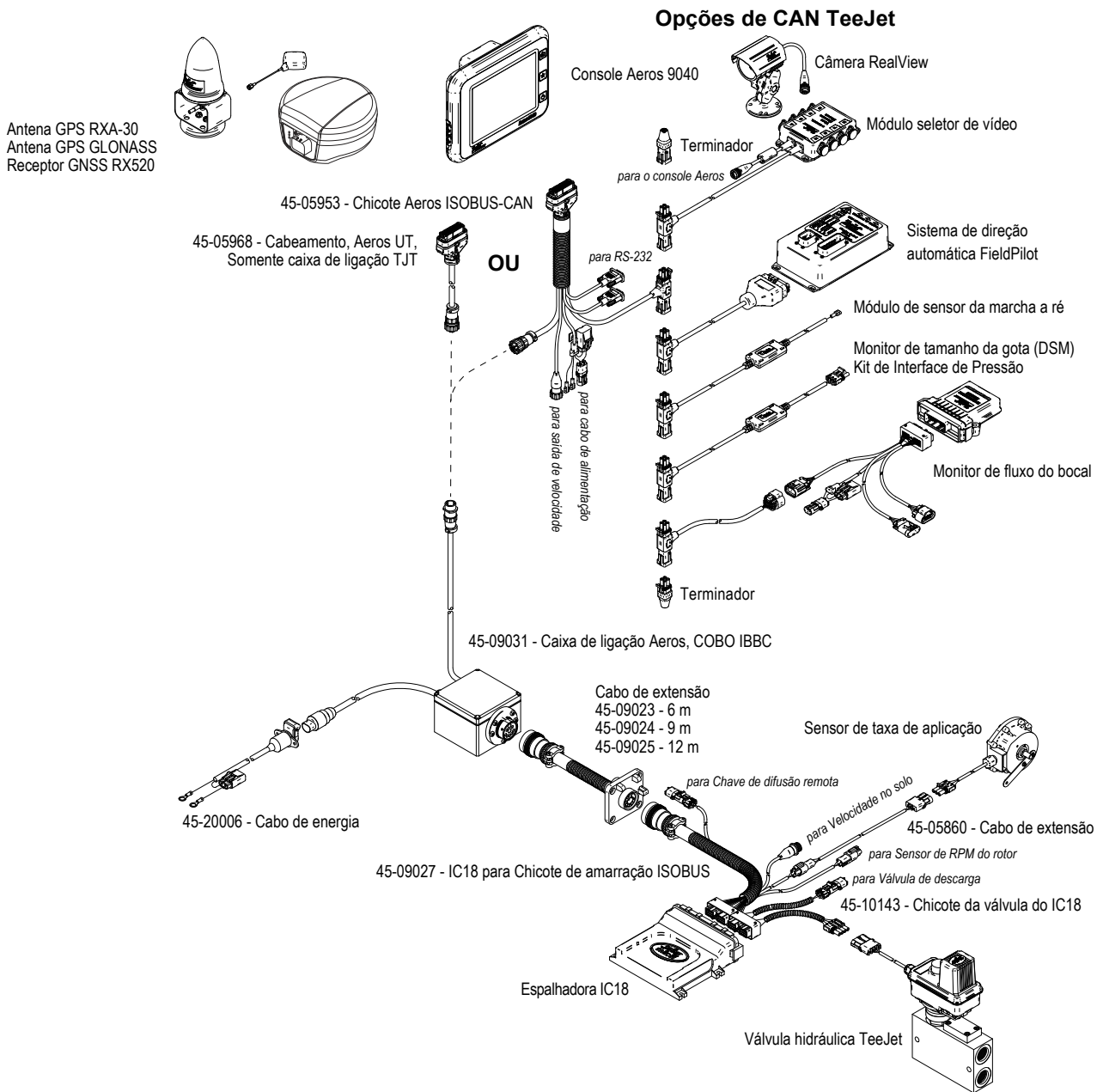
Figura 35: Espalhadora Aeros IC18
