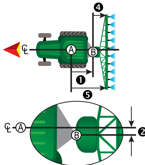
Figura 31: Montagem traseira
