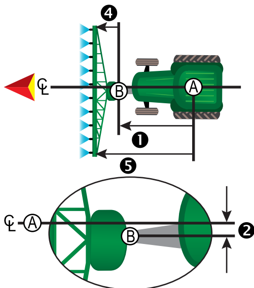
Figura 30: Montagem frontal
