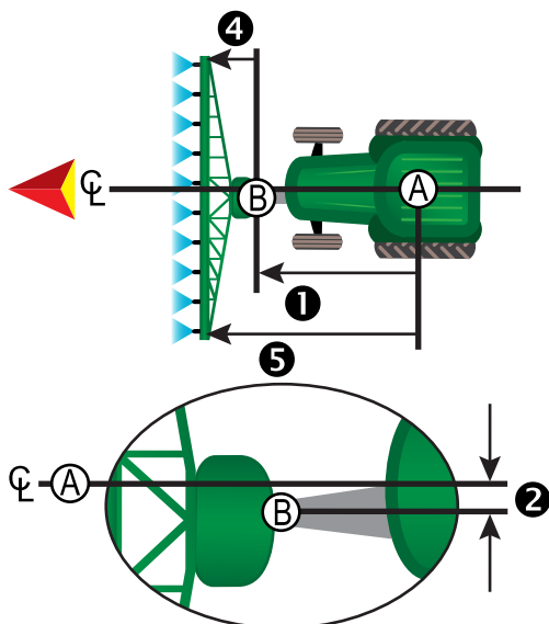
Figure 30 : Montage avant
