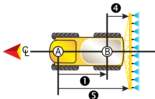
Figure 29 : Montage arrière
